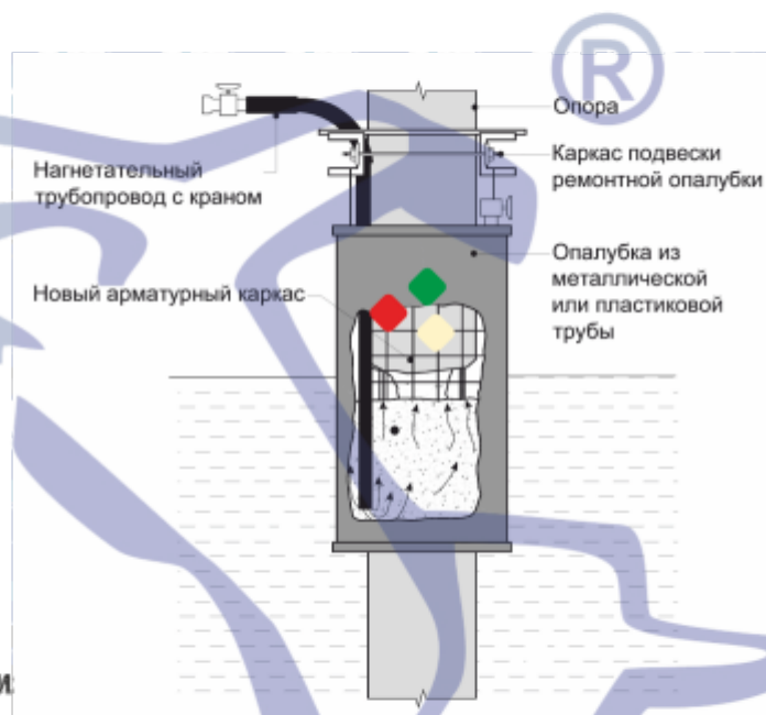
Схема ремонта в подводных условиях с помощью устройства накладной манжеты (подвеска опалубки над уровнем воды) 6
