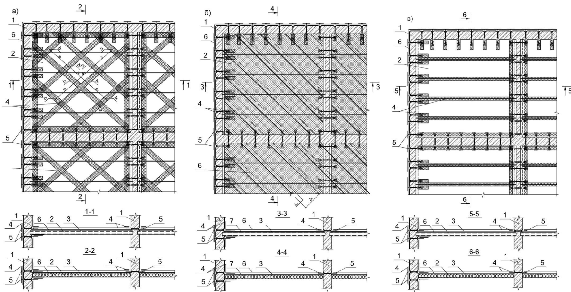
а) отдельными диагональными углеродными однонаправленными лентами; б) сплошной углеродной двунаправленной тканью; в) отдельными полосами углеродно двунаправленной ткани 1 – кирпичная стена; 2 – плиты перекрытия; 3 – конструкция пола; 4 – углеродные однонаправленные ленты; 5 – углеродные анкерные жгуты; 6 – ремонтный состав
