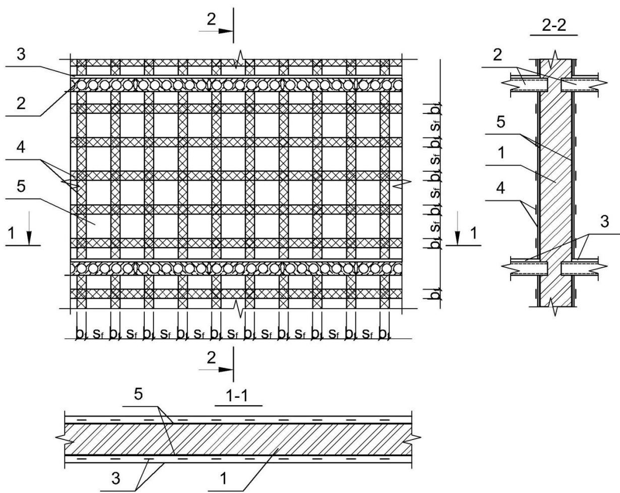
1 – стена; 2 – плиты перекрытия; 3 – конструкция пола; 4 – углеродные однонаправленные ленты; 5 – ремонтный состав Рисунок 4.1 – Усиление стен путем наклейки вертикальных и/или горизонтальных углеродных однонаправленных лент
