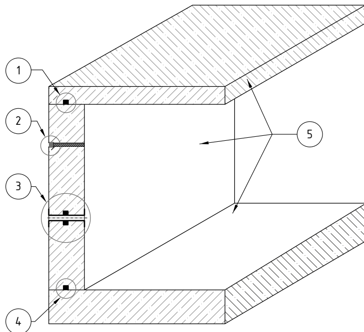
Рисунок 9.1 — Общая схема гидроизоляции строительных конструкций при монолитном строительстве. Обозначения: 1. Гидроизоляция швов бетонирования (п. 9.2); 2. Гидроизоляция технологических отверстий (п. 9.4); 3. Гидроизоляция гильзы для ввода инженерных коммуникаций (п. 9.3); 4. Гидроизоляция швов бетонирования (п. 9.2); 5. Гидроизоляция ограждающих конструкций (п. 9.1).
