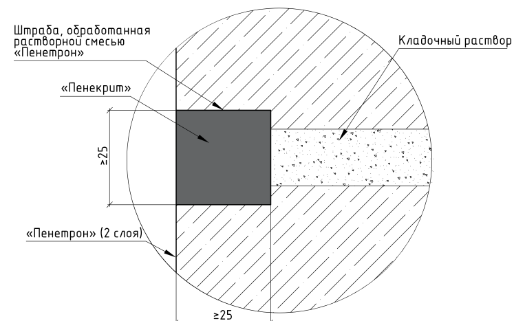
Рисунок 8.4 — Схема гидроизоляции шва между бетонными блоками (ФБС)
