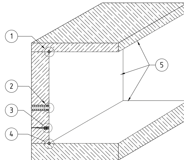
Рисунок 8.1 — Общая схема гидроизоляции существующих строительных конструкций. Обозначения: 1. Гидроизоляция статических швов и трещин (п. 8.3); 2. Гидроизоляция инженерных коммуникаций (п. 8.5); 3. Ликвидация течей (п. 8.4); 4. Гидроизоляция статических швов и трещин (п. 8.3); 5. Гидроизоляция ограждающих конструкций (п. 8.2).
