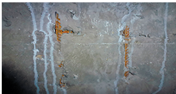
Недостаточная толщина защитного слоя
