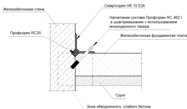
Рис. 2 Дюуплотнение шва/трещины шовным материалом
